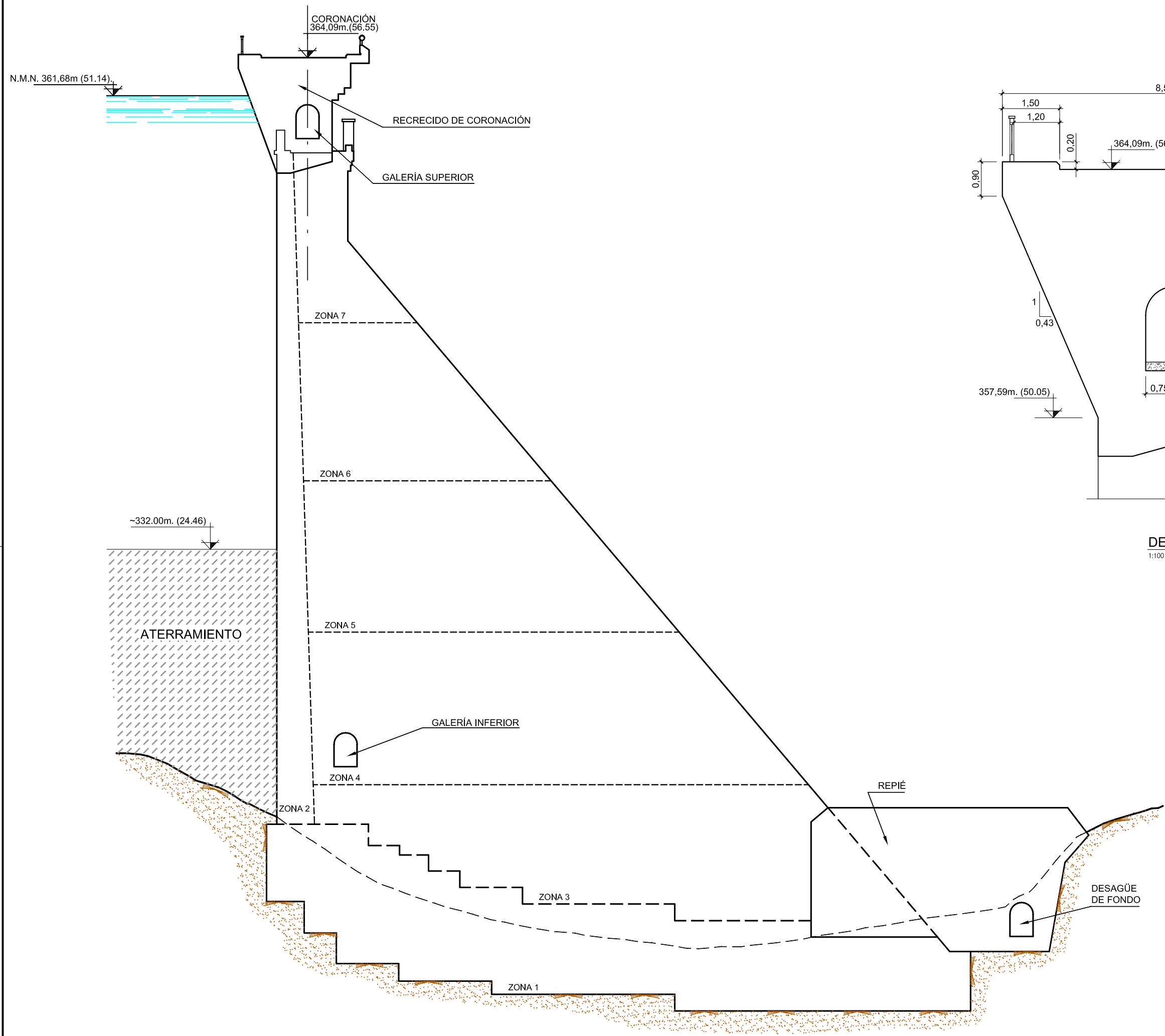
SECCIÓN TIPO 1:250
