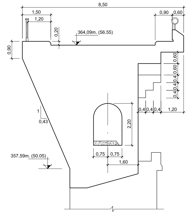
DETALLE CORONACIÓN 1:100
