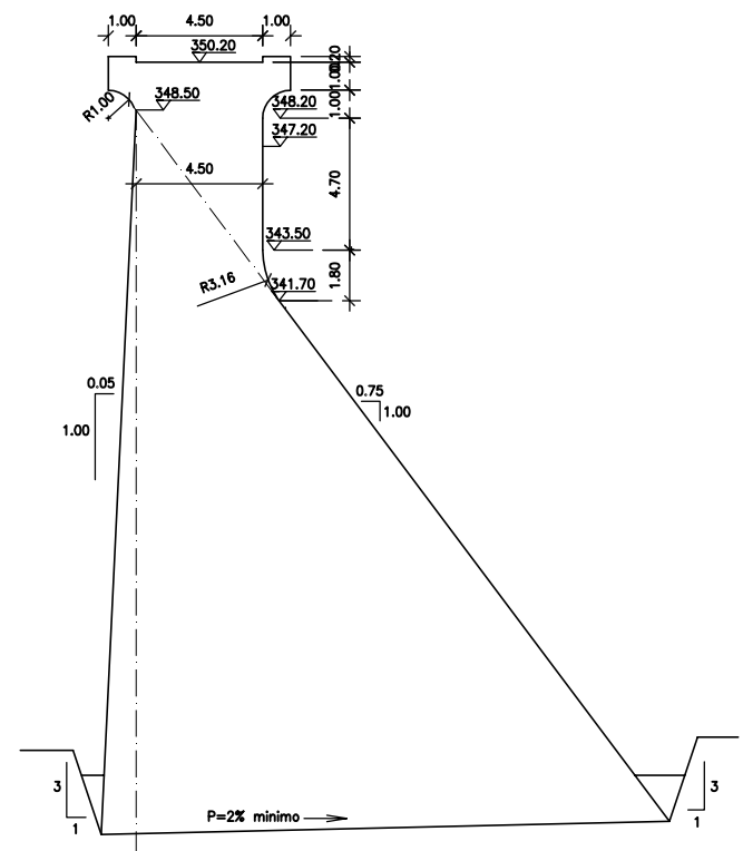
SECCION TIPO POR ESTRIBOS
