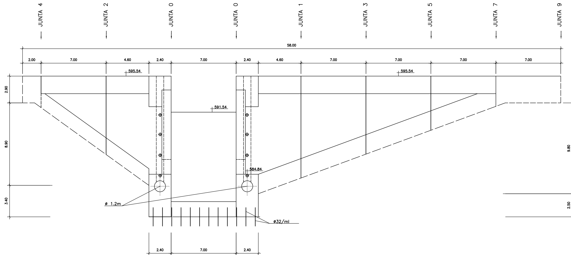
ALZADO VISTO DESDE AGUAS ABAJO ESCALA 1:100
