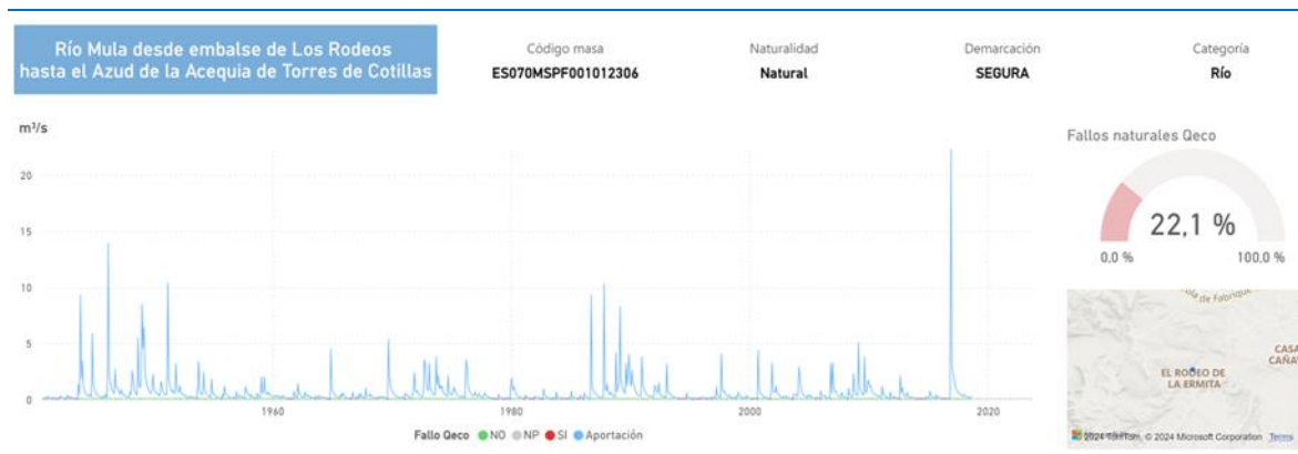
Figura 11. Ejemplo de comparación del régimen de caudales no alterados con los caudales mínimos
