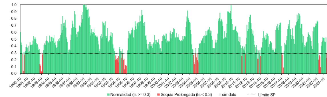
Figura 3. Evolución del índice global de demarcación para la sequía prolongada en el periodo 1980/81 - 2023/24.
