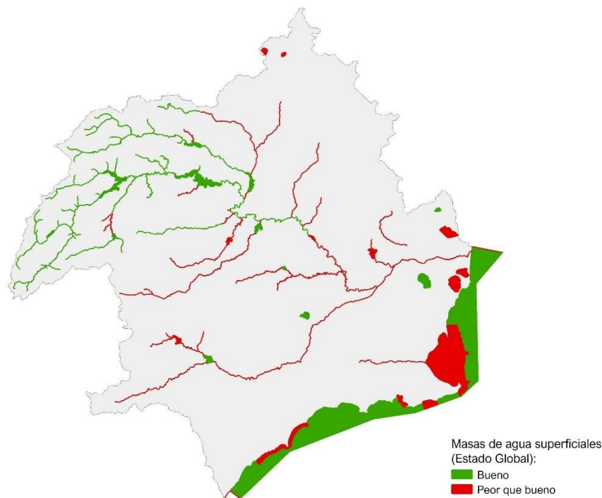
Figura 6. Estado de las masas de agua superficial
