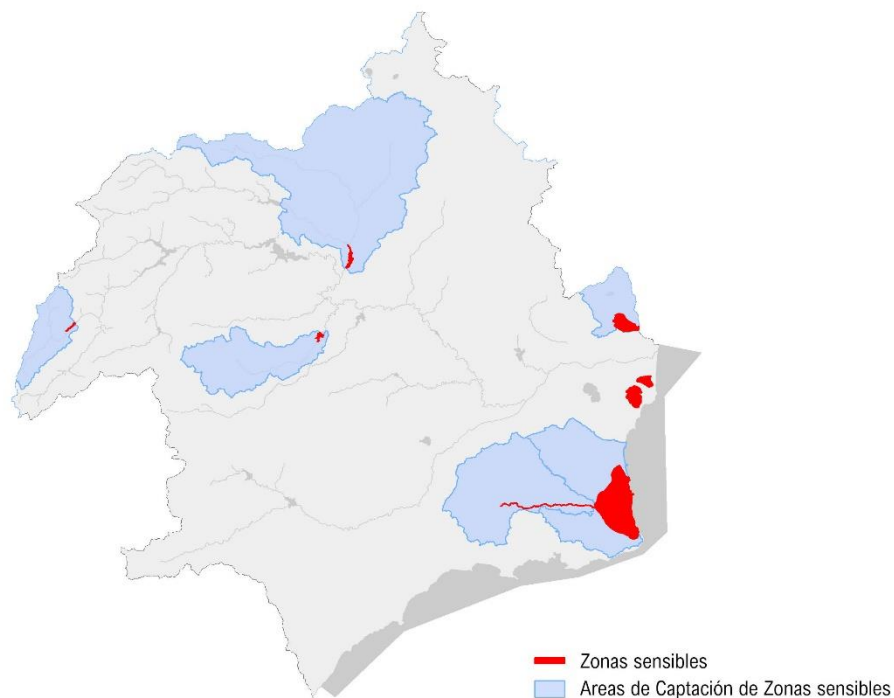
Figura 8. Zonas sensibles en la Demarcación Hidrográfica del Segura
